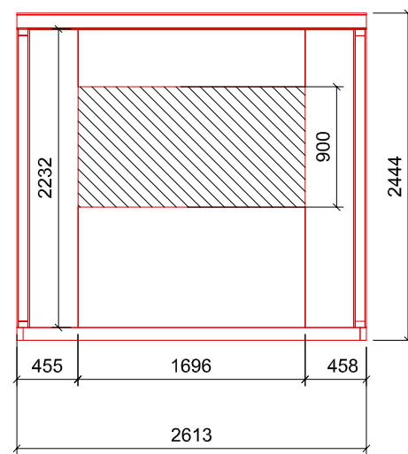
Font Elevation
