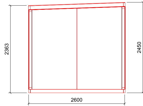
LH Elevation
