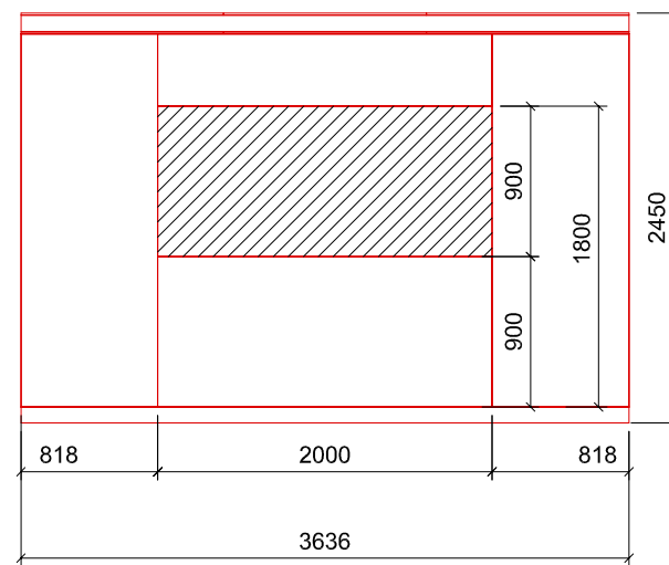
Font Elevation
